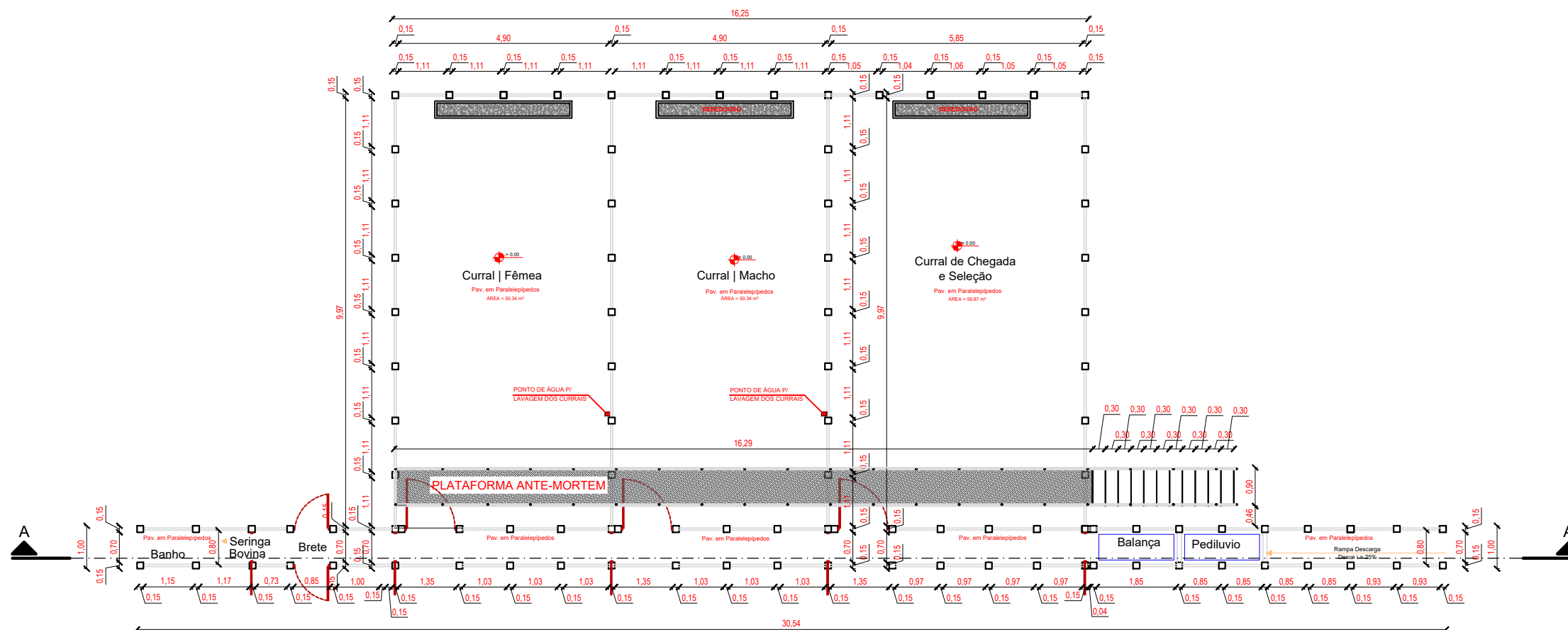
PLANTA BAIXA _ CURRAL ESCALA _____ 1/125
